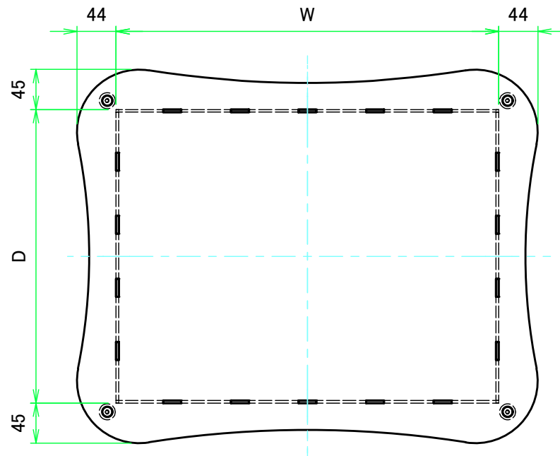
上カバー / Top cover
